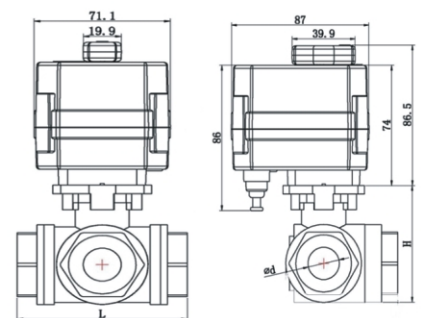
三通式
