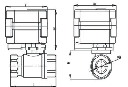
两通式
